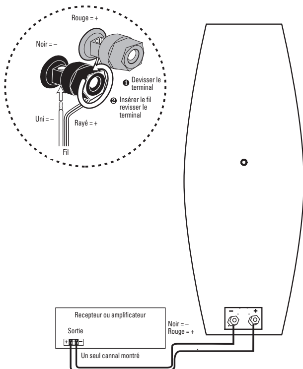
Figure 3. Le schéma de câblage indique les connexions de polarité pour un canal d'un système de cinéma à domicile.
